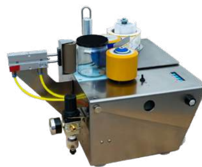
Edykedy mit Pneumatik-Rückwand für die stehende Etikettierung
