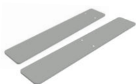
Bodenplatte für mittlere Formate 400 x 100 x 8 mm Bohrung mittig oder hinten erhältlich Zubehör-Nr. 10
